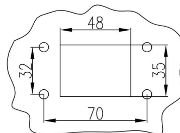
面板开孔图
